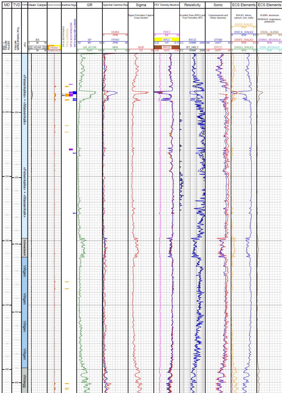
Fig. 3-2: Main logs of the composite dataset in the «Felsenkalke» + «Massenkalk» to the Wildegg Formation
